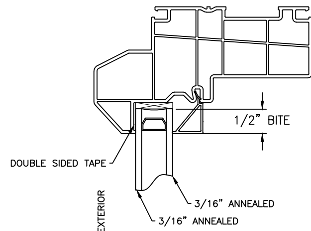
IG GLAZING GL1
